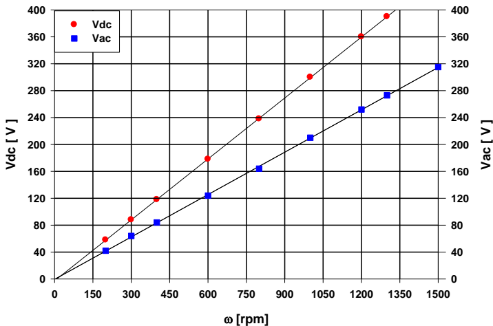
No-Load
